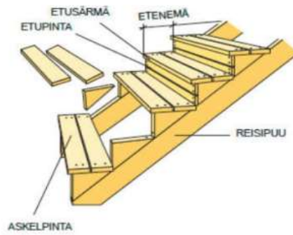
KUVA 3. Yleinen porrask rakenne
